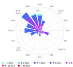
Rose des vents (direction d'où vient le vent) En décembre 2020 à Site
