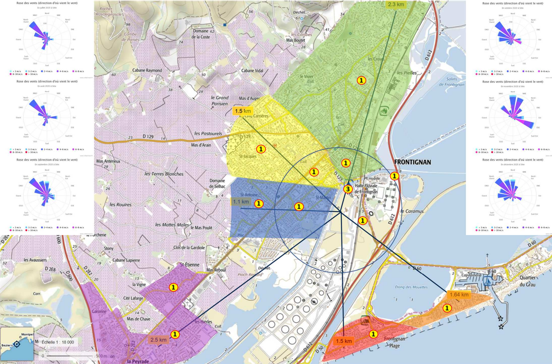
Rose des vents (direction d'où vient le vent) En octobre 2020 à Site
