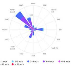
Rose des vents (direction d'où vient le vent) En septembre 2020 à Site
