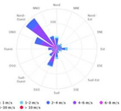
Rose des vents (direction d'où vient le vent) En août 2020 à Site
